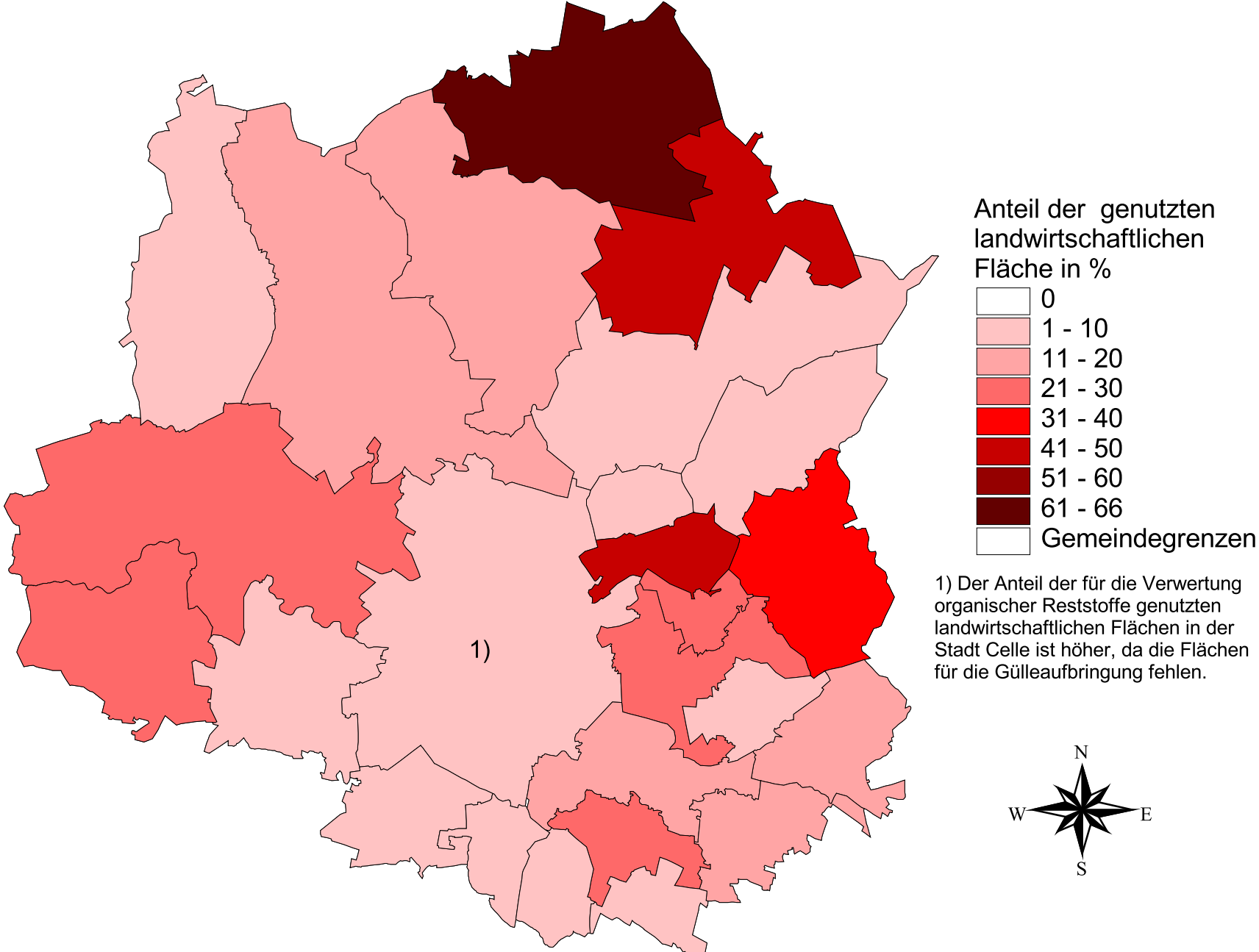
D 3.2 Abb.8: Anteil der für die Verwertung organischer Reststoffe (Klärschlamm, Gülle) genutzten landwirtschaftlichen Flächen in den Gemeinden im Jahr 2002
